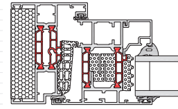
58BW FLUSH HI JAMB
